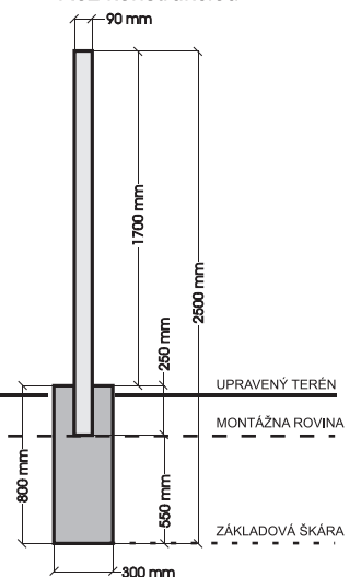
Rez konštrukciou
